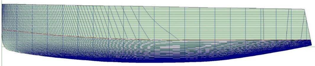
Rys. 1. Widok przykładowego kadłuba łodzi
