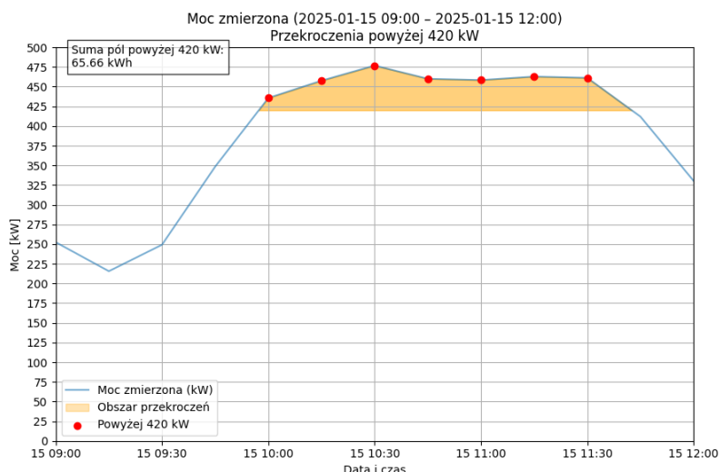
Rys. 17. Okres przekroczenia mocy zamówionej, zarejestrowany w dniu 15.01.2025
